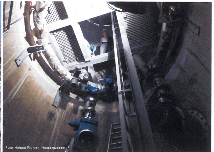
Blick von der Schachtsohle zur Ringleitung
