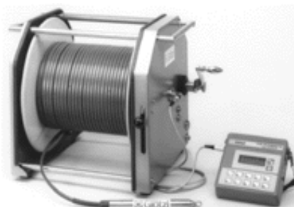
Beispiel eines Glötzl-Systems
