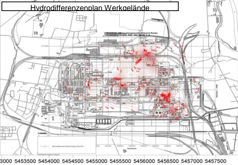
Benzolverteilung 2005 Werkgebiets
