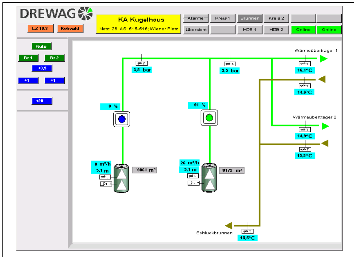
Funktionsbild der Grundwasserfassungsanlage der ZKV Wiener Platz
