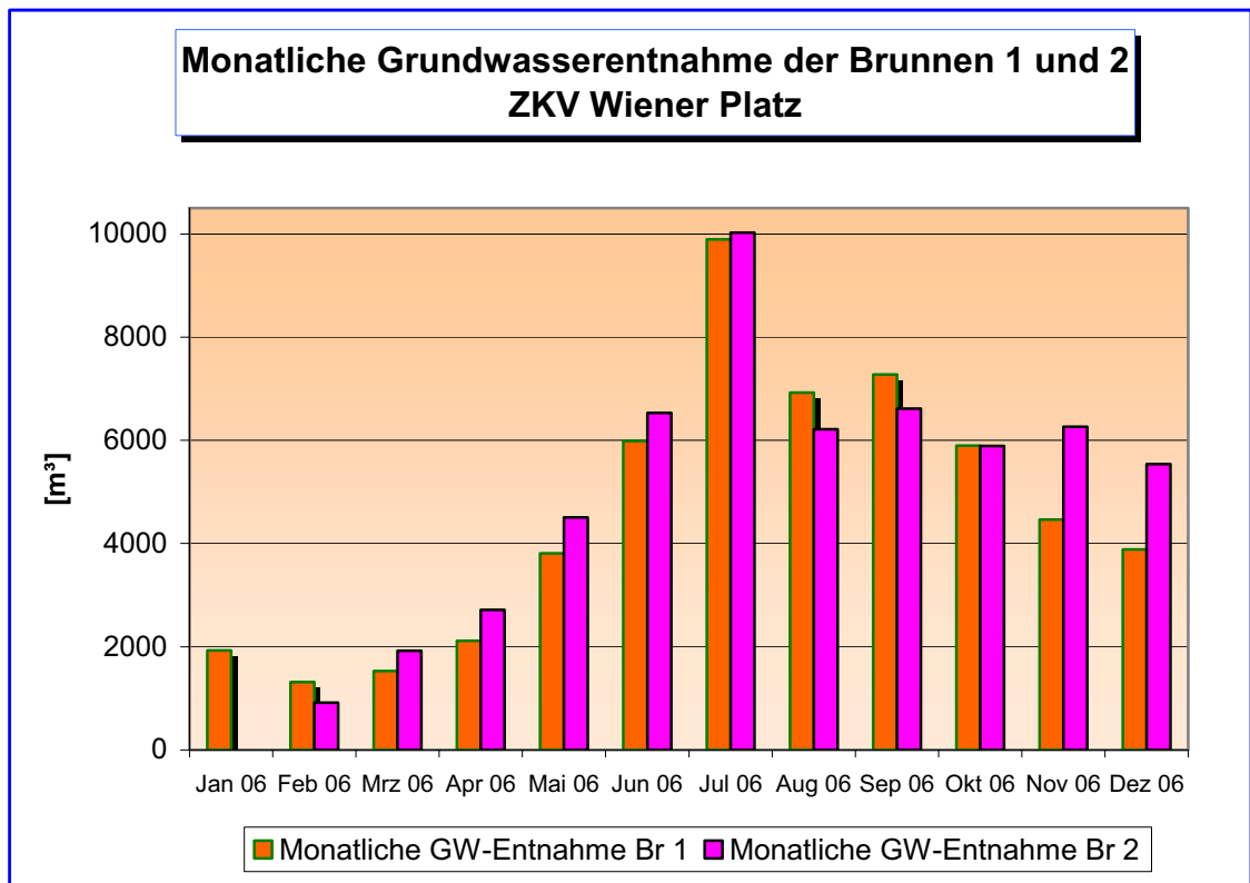
Detailauswertung Fördermenge beider Brunnen
