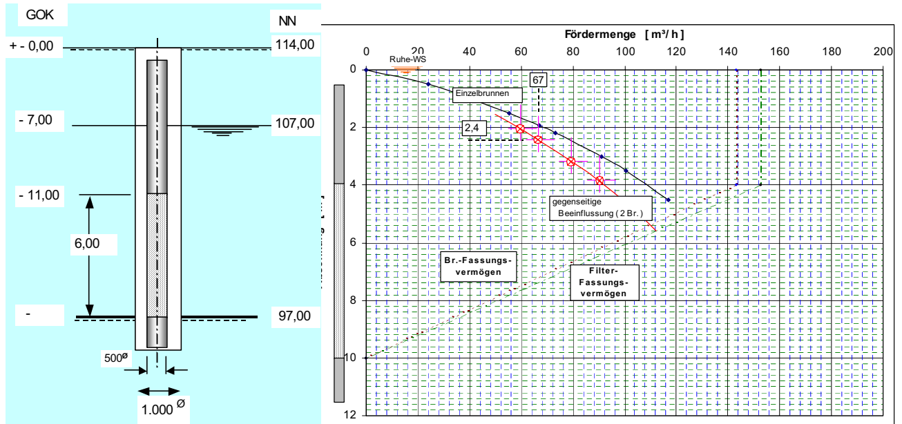
Prinzipskizze der Entnahmehrunden mit Darstellung des Ruhewasser-Spiegels und der Absenkberechnung bei 60 m 3 /h (ca. 2 m).
