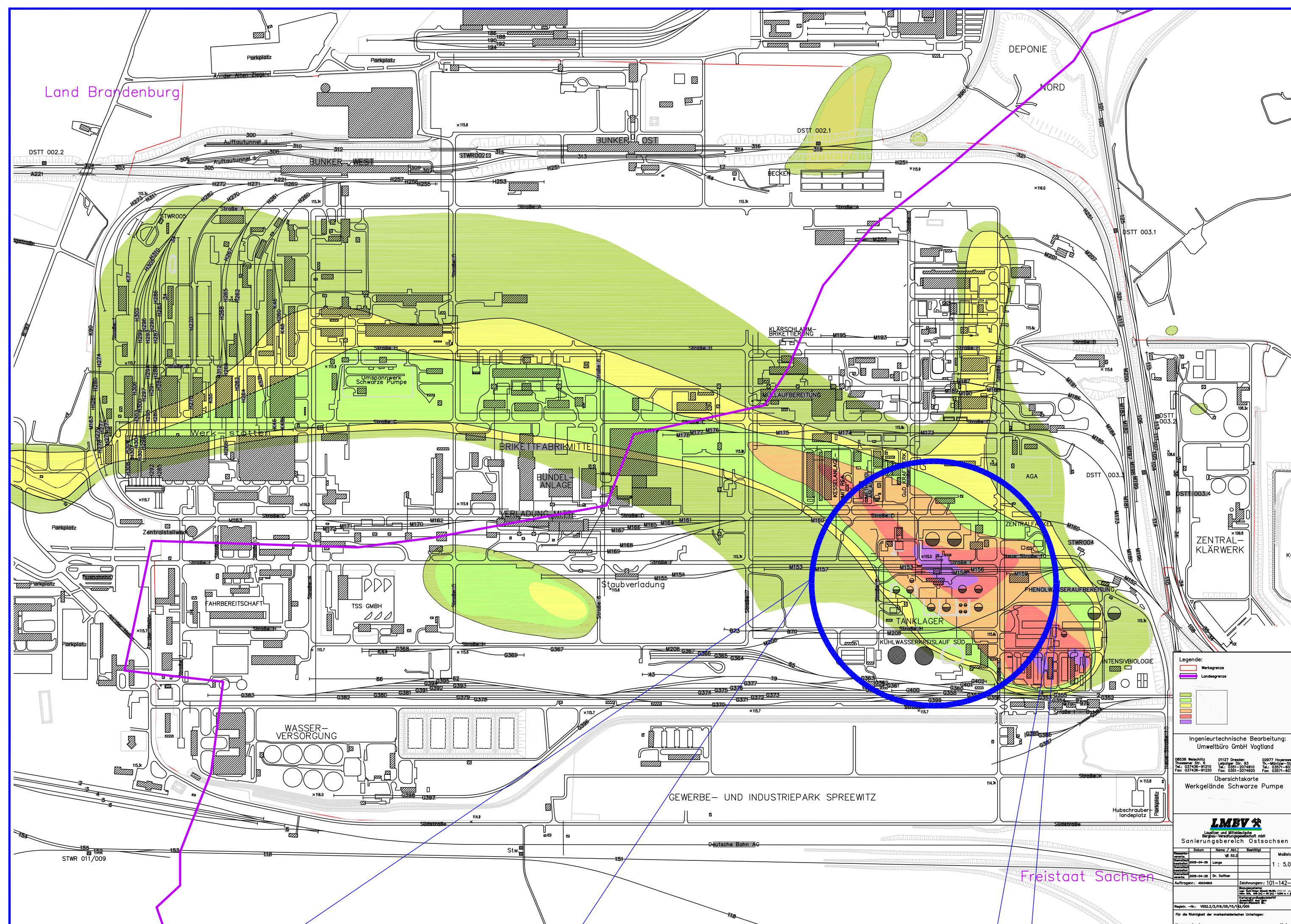
Übersichtskarte mit Benzolverteilung 2004 auf dem Werkgelände Schwarze Pumpe
