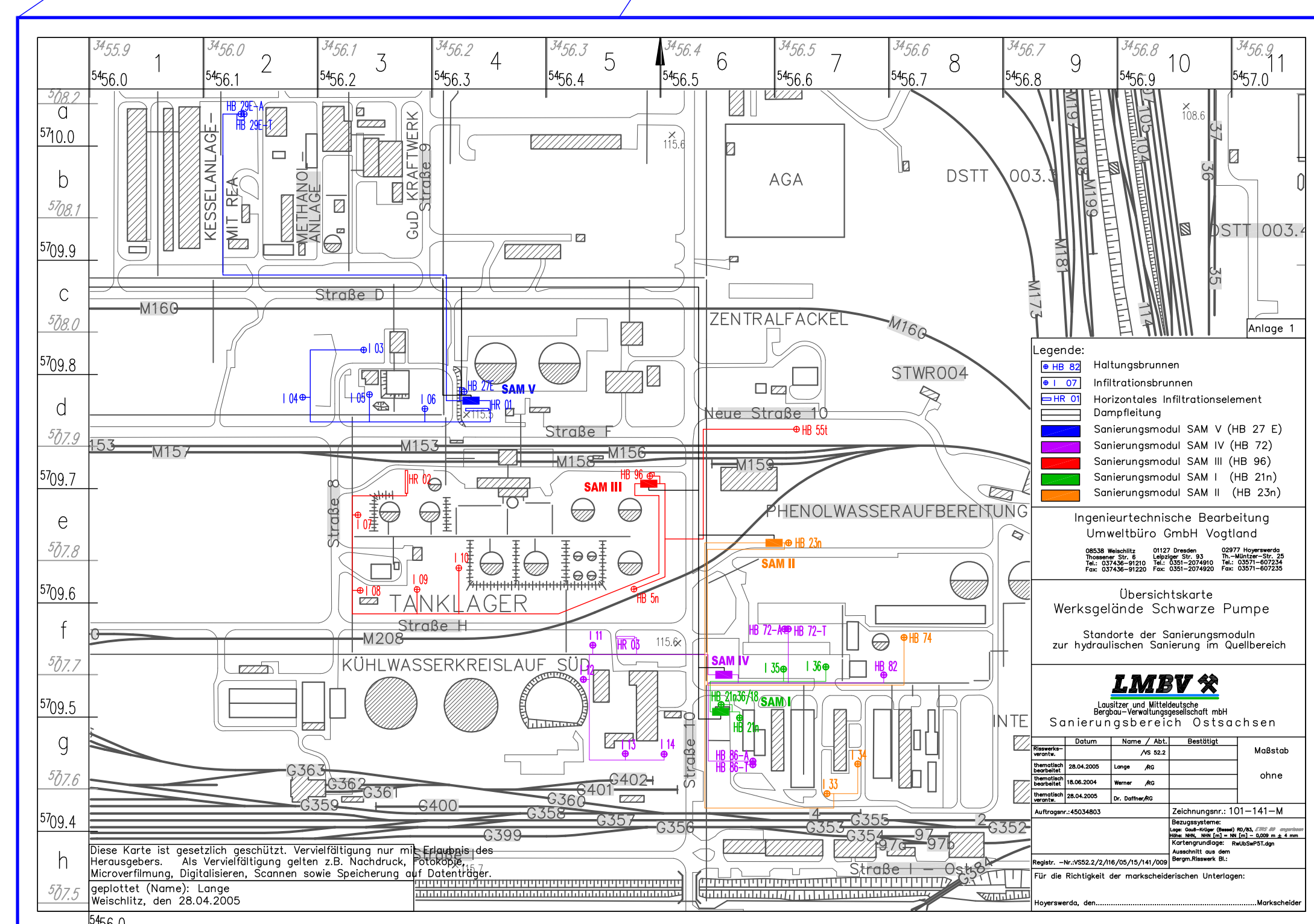
Übersicht der im Betrieb befindlichen Sanierungsmodule (MPPE-Anlage)
